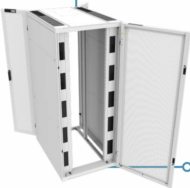
Das Dach hat links, rechts und in der Mitte Aussparungen, die mit Bürstenleisten und Abdeckblenden abgedeckt sind.
