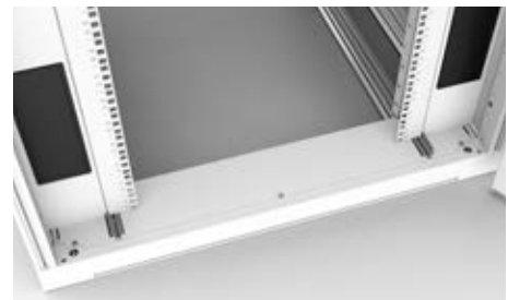
Paket für Luftstrom-Management unten am 800 mm breiten Schrank
