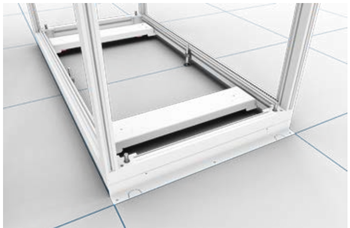
Einfache Ausrichtung an Bodenfliesen durch Wendesockel
